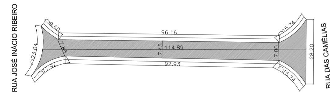
2 DETALHAMENTO DA RUA DAS HORTÊNCIAS ESC.: 1:100
