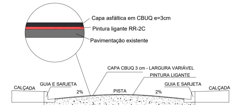
6 CORTE TRANSVERSAL RECAPE SEM ESCALA
