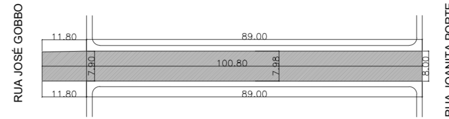
4 DETALHAMENTO DA RUA LEONIDAS ROMANO DA SILVA ESC.: 1:100
