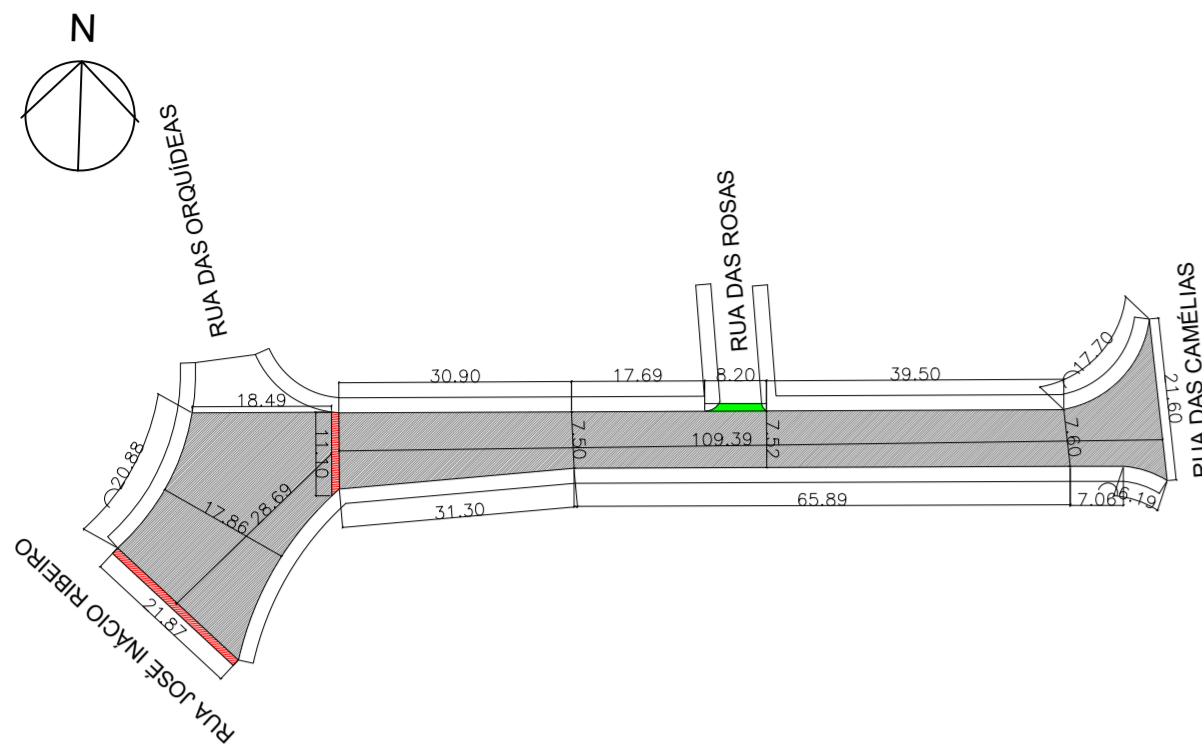
1 DETALHAMENTO DA RUA DAS MARGARIDAS ESC.: 1:100
