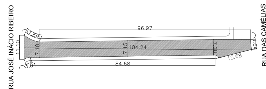
3 DETALHAMENTO DAS RUAS DAS TULIPAS ESC.: 1:100
